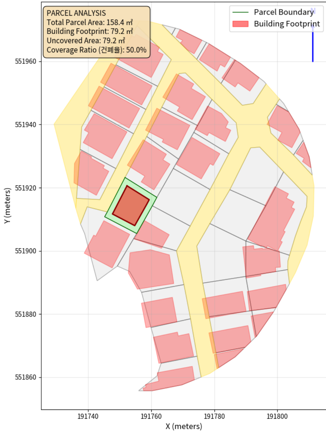
대지 배치도 (원본)
